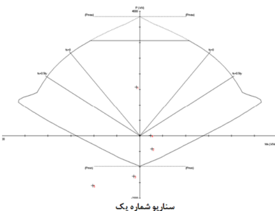
شکل ۱۲- ظرفیت مقطع پوشش نهایی و نیروهای القا شده به آن
