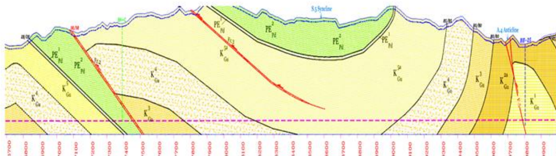
شکل ۱- نمایی از یک برش زمین‌شناسی و مسیر حفر تونل (Ramezannia et al., 2015)
