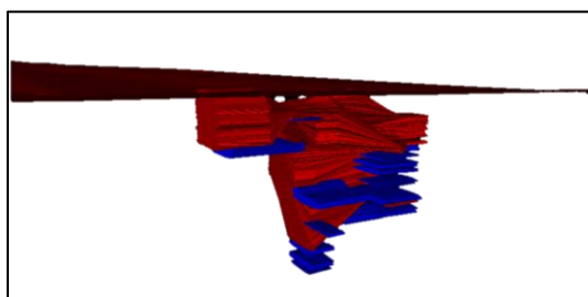
شکل ۴- مدل سه‌بعدی تهیه شده برای بخش شمال شرقی آنومالی ۱۲ (Jabinpoor et al., 2015)
