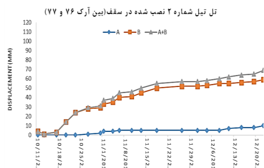
شکل ۱۵- نمودار جابجایی نقاط جابجایی سنج شماره ۲
