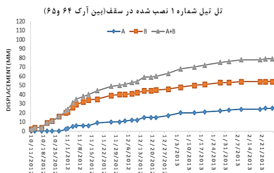
شکل ۱۴- نمودار جابجایی نقاط جابجایی سنج شماره ۱
