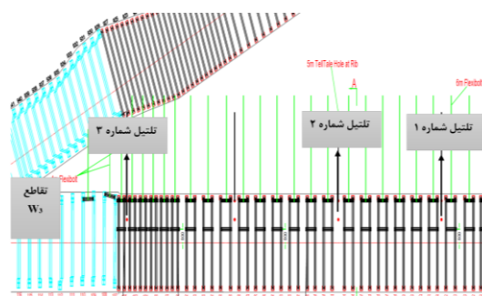
شکل ۱۳- محل نصب جابجایی‌سنج‌ها در اطراف تقاطع W_3
