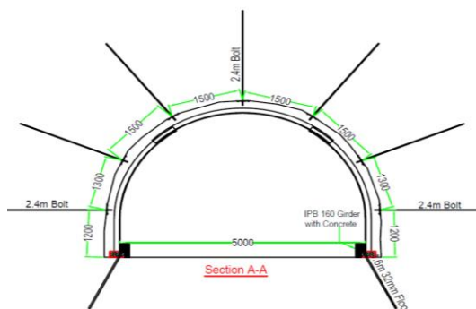
شکل ۳- آرک کشویی V_{29} و پیچ‌سنگ‌ها در مقطع نعل‌اسبی
