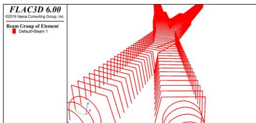
شکل ۱۰- نمایی از قاب‌های IPB مدل‌سازی شده در تقاطع W3
