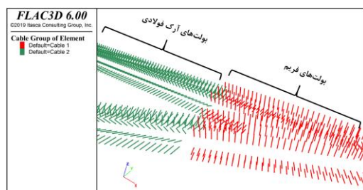
شکل ۱۱- نمایی میل‌مهاری مدل‌سازی شده در تقاطع W3
