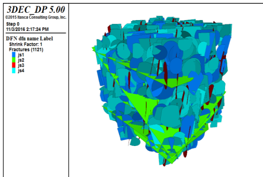
شکل ۵- مدل DFN متشکل از ۱۱۲۱ درزه در بلوک ۱۰ مترمکعبی
