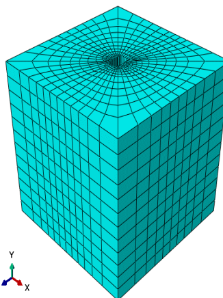
شکل ۱- نحوه‌ی مش بندی خاک (Farshidi, 2023)
