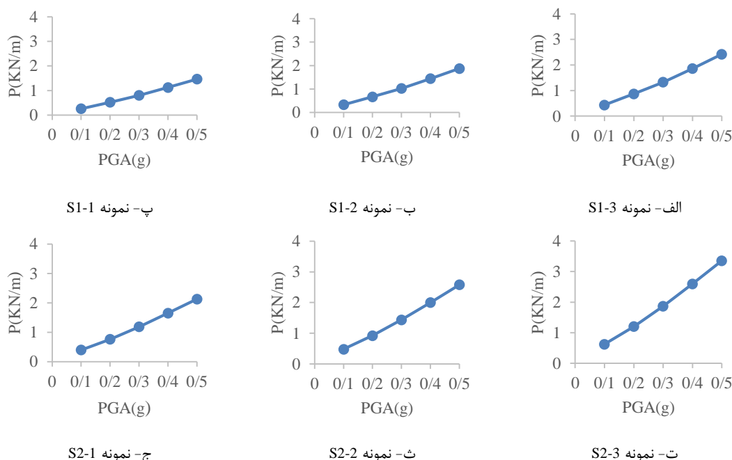
شکل ۱۰- نمودار مقدار بار زلزله‌ی محاسبه شده برای نمونه‌های مورد بررسی (Farshidi, 2023)
