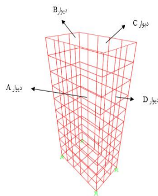
شکل ۱۲- نمونه‌ی شفت مدل شده در SAP2000
