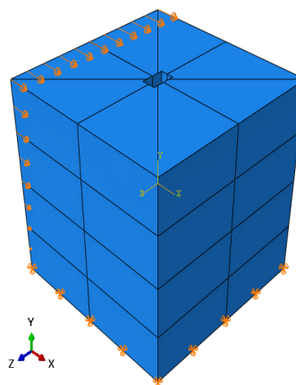
شکل ۲- نحوه‌ی اعمال تغییرمکان مثلثی اجباری (Farshidi, 2023)
