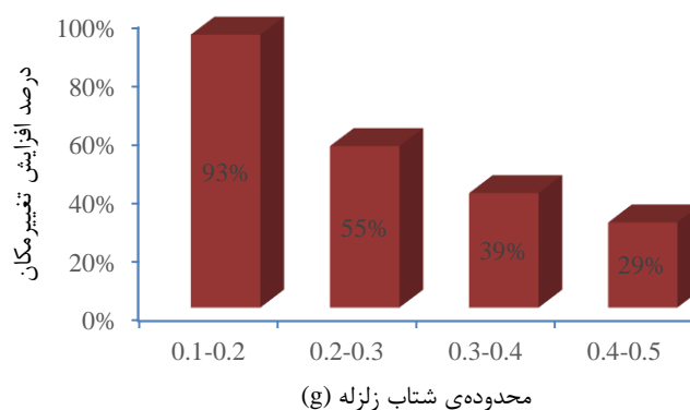
شکل ۱۵- درصد افزایش تغییرمکان در اثر افزایش شتاب زلزله برای نمونه‌ی S2 (Farshidi, 2023)
