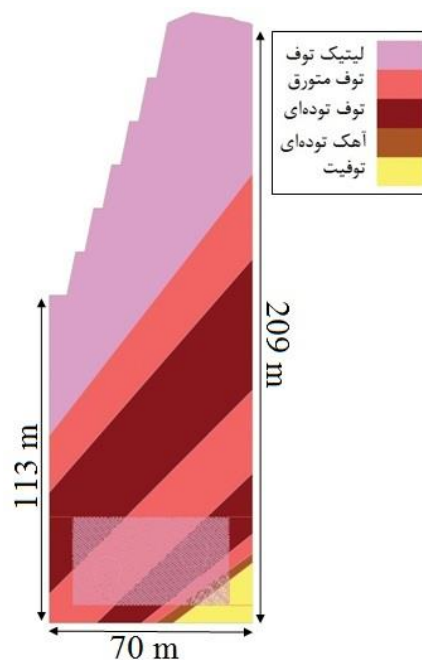
شکل ۴- مدل‌سازی هندسی وضعیت لایه‌بندی در مقطع
