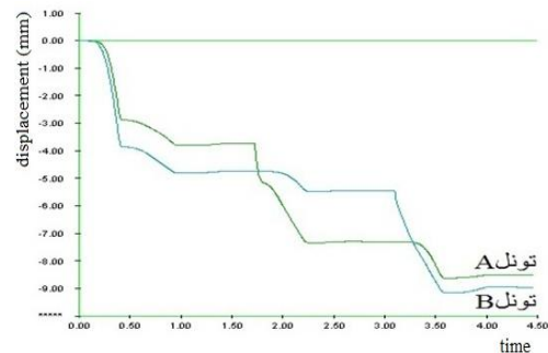
شکل ۶- جابجایی‌های قائم سقف تونل‌های انحراف آب سد مشمیا زنجان طی مراحل حفاری
