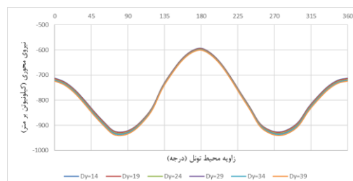
شکل ۱۴- نیروی محوری (خط اتصال قائم - غیر هم زمان)
