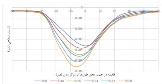
شکل ۱۶- نشست سطحی (خط اتصال مایل - غیر هم زمان)
