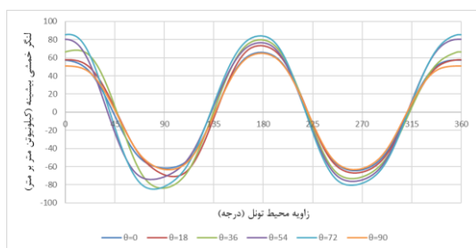
شکل ۱۸- لنگر خمشی (خط اتصال مایل - غیر هم زمان)
