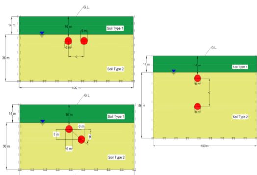
شکل ۲- هندسه مدل‌های ساخته شده
