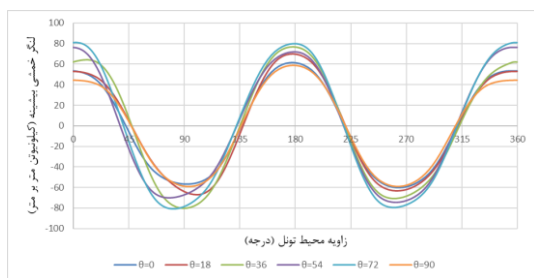
شکل ۱۷- لنگر خمشی (خط اتصال مایل - هم زمان)
