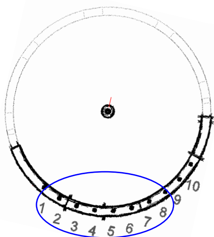
ب- نمایش قرارگیری جک‌ها در قطعات کف
