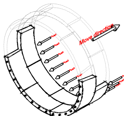
الف- نمایش سه بعدی از وضعیت قرارگیری قطعات
