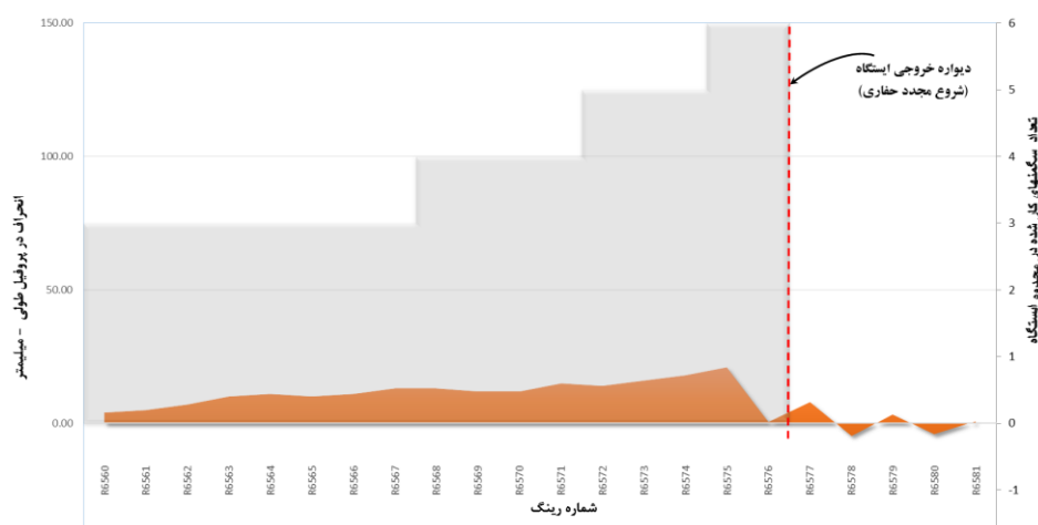
شکل ۱۴- میزان ثبت‌شده انحراف دستگاه در ایستگاه 16 خط ۶ مترو تهران
