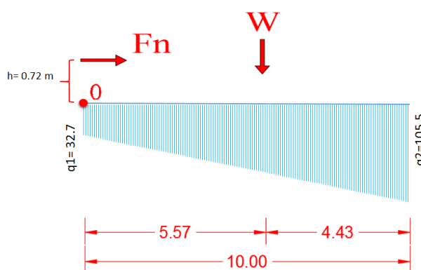
شکل ۶- نمایش مقدار نیروهای عکس‌العمل در طول ایستگاه
