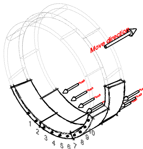
الف- نمایش سه بعدی از وضعیت قرارگیری قطعات کف
