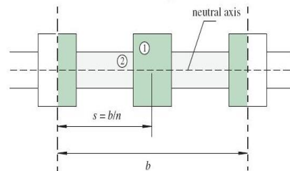
الف) نمایش شماتیک یک مقطع عرضی از لایه نگه‌دارنده شامل مواد مختلف ۱ و ۲
