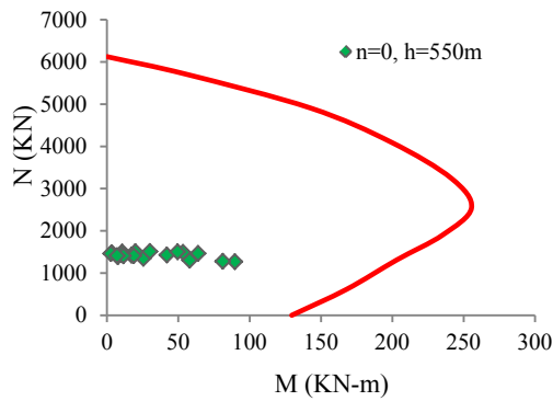
شکل ۲۲- بررسی پایداری سازه‌ای پوشش یکپارچه در محدوده‌ی باربره‌ی ۵۵۰ متر
