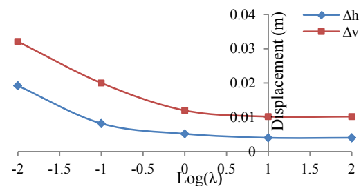
شکل ۹- جابجایی پوشش تونل با مقدار سختی مفصل
